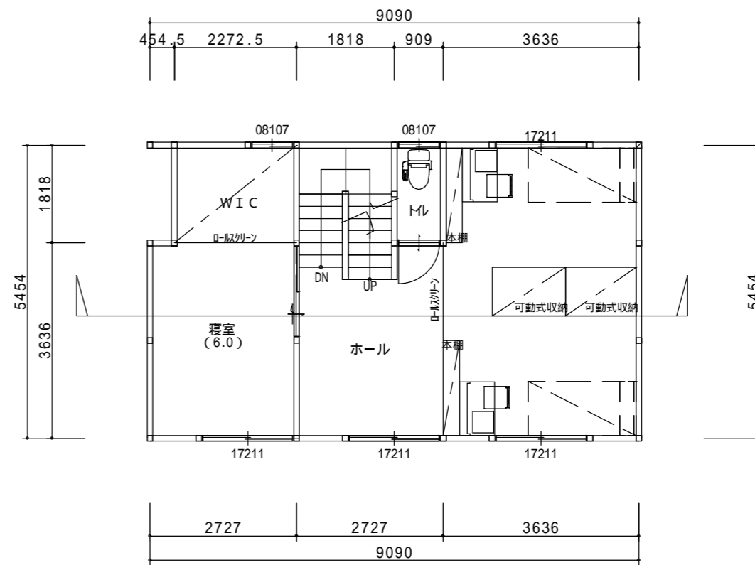
2階平面図
