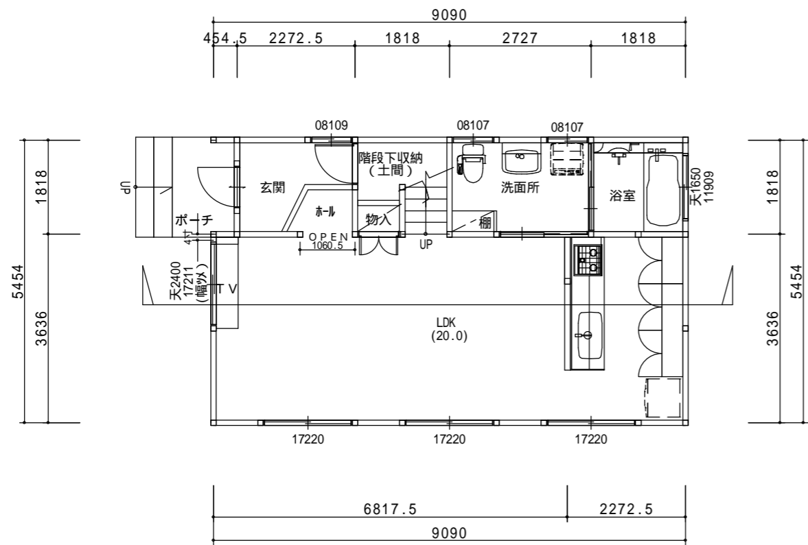
1階平面図
